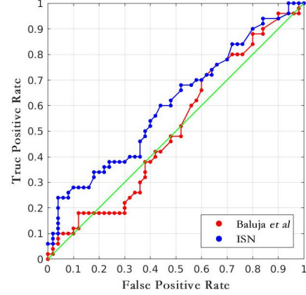
图 9. [5] 和 ISN 生成的载密图像在 StegExpose [7] 设置不同阈值下检测获得的 ROC 曲线。
