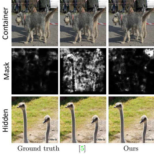
图 8. 伪造检测。第二行中的 Mask 分别是第一行中载密图像由 ManTra-Net [57] 检测的结果。第三行是隐藏图像。
